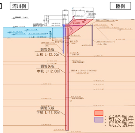
施工断面
