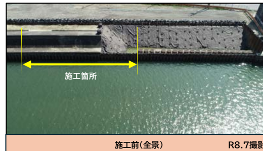
施工前(全景)
