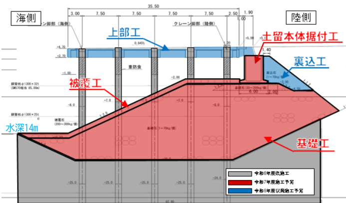
【岸壁標準断面図】
