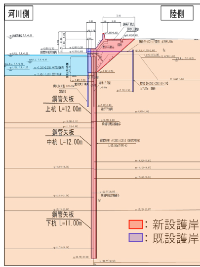
標準護岸断面図
