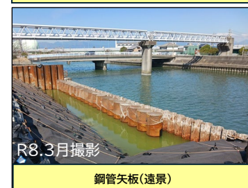
鋼管矢板(遠景)
