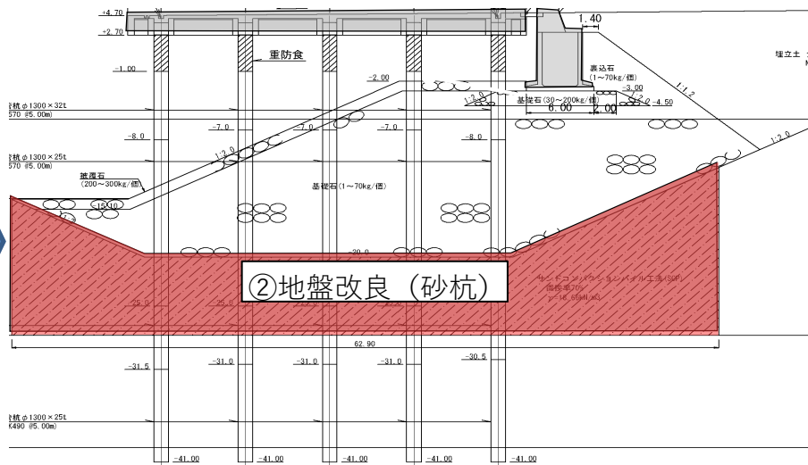
標準断面図
