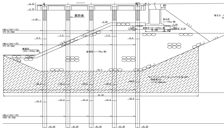
標準断面図
