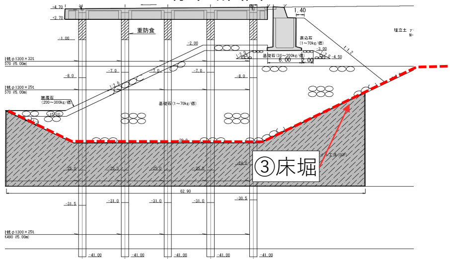
標準断面図
