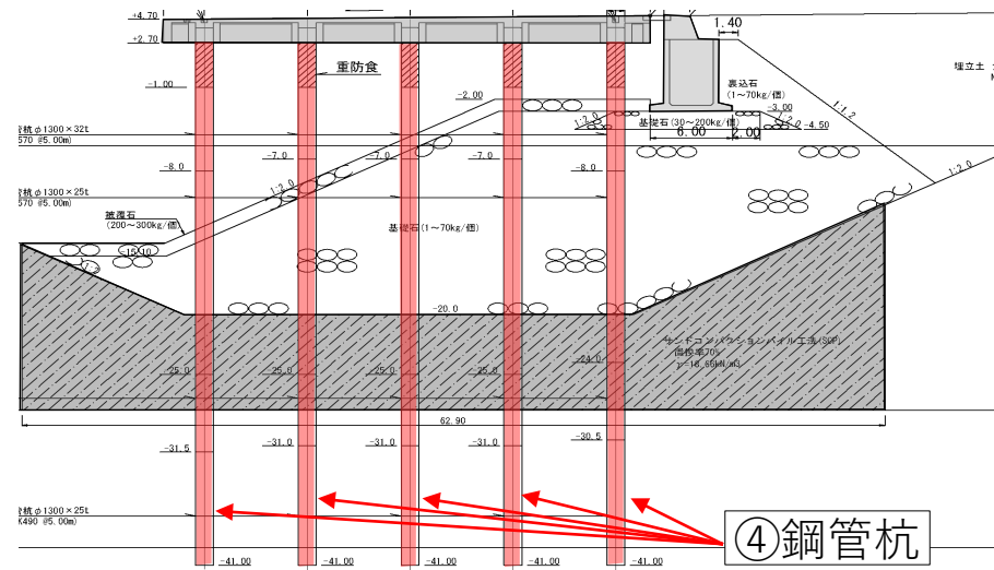
標準断面図
